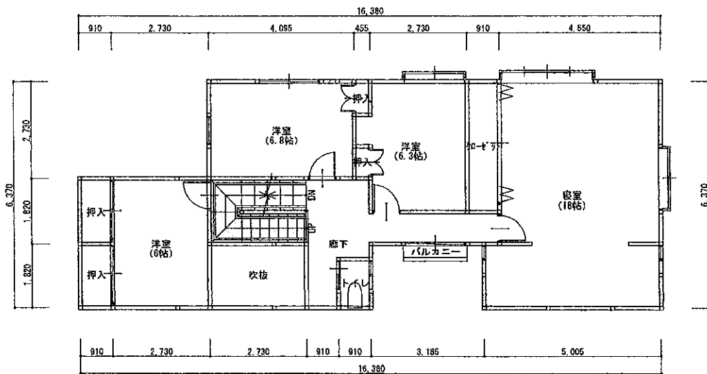
2階 平面図 S:1/100
